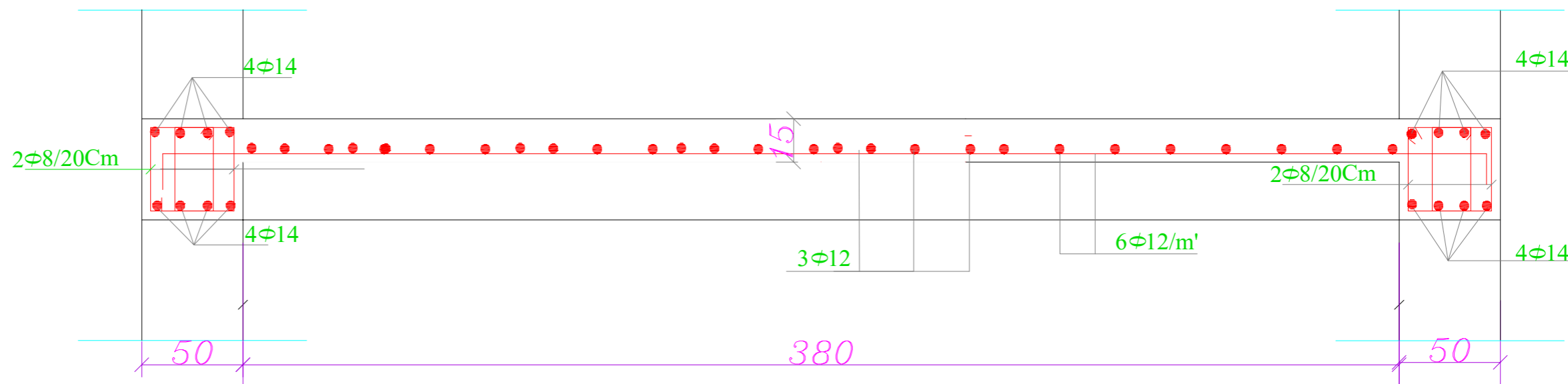
مقطع في بلاطة سقف الغرفة وارضية الغرفة
