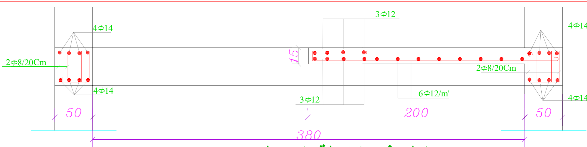
مقطع في البلاطة الوسطى
